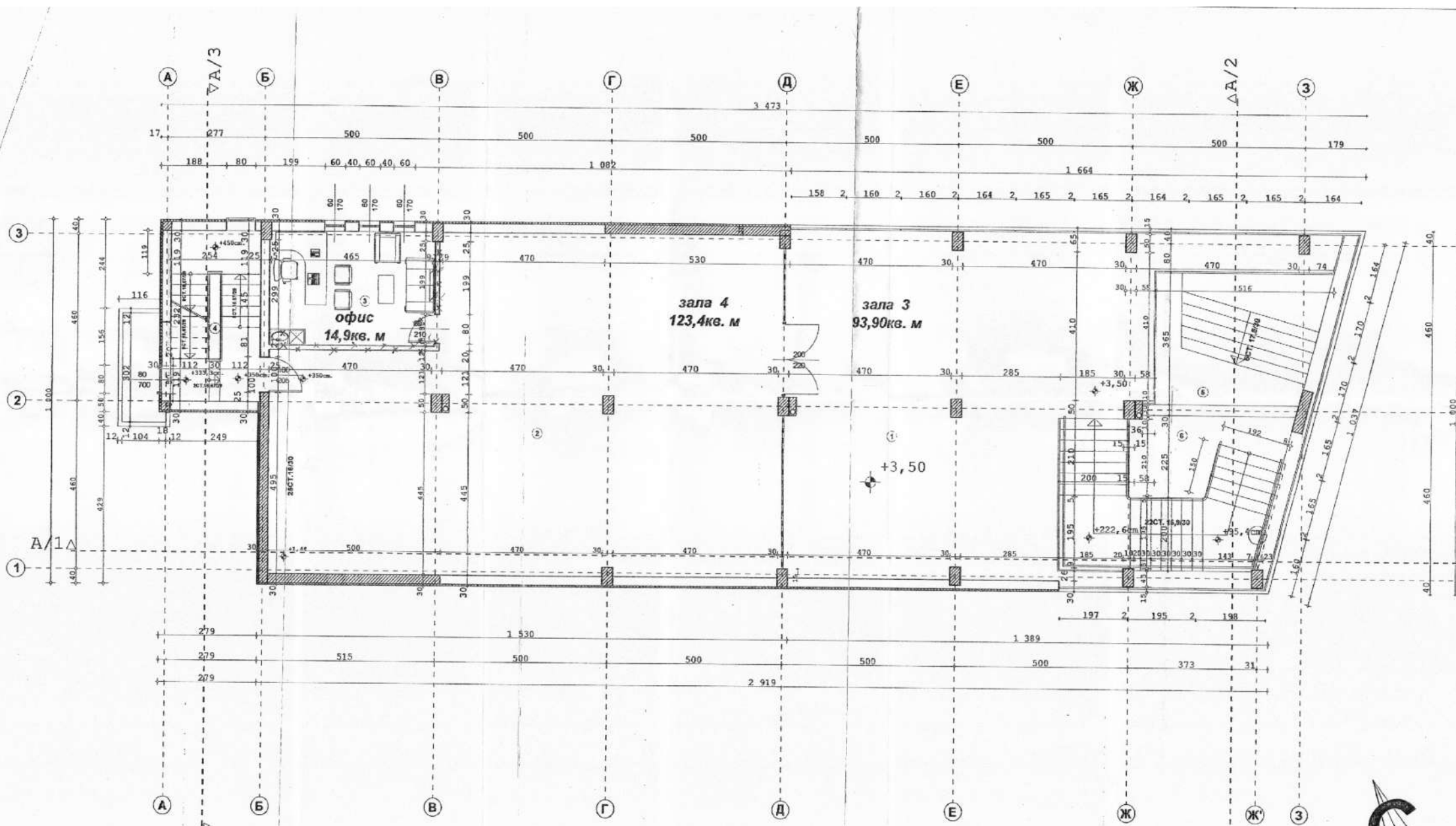
Разпределение на кота +3,50 М 1:50
