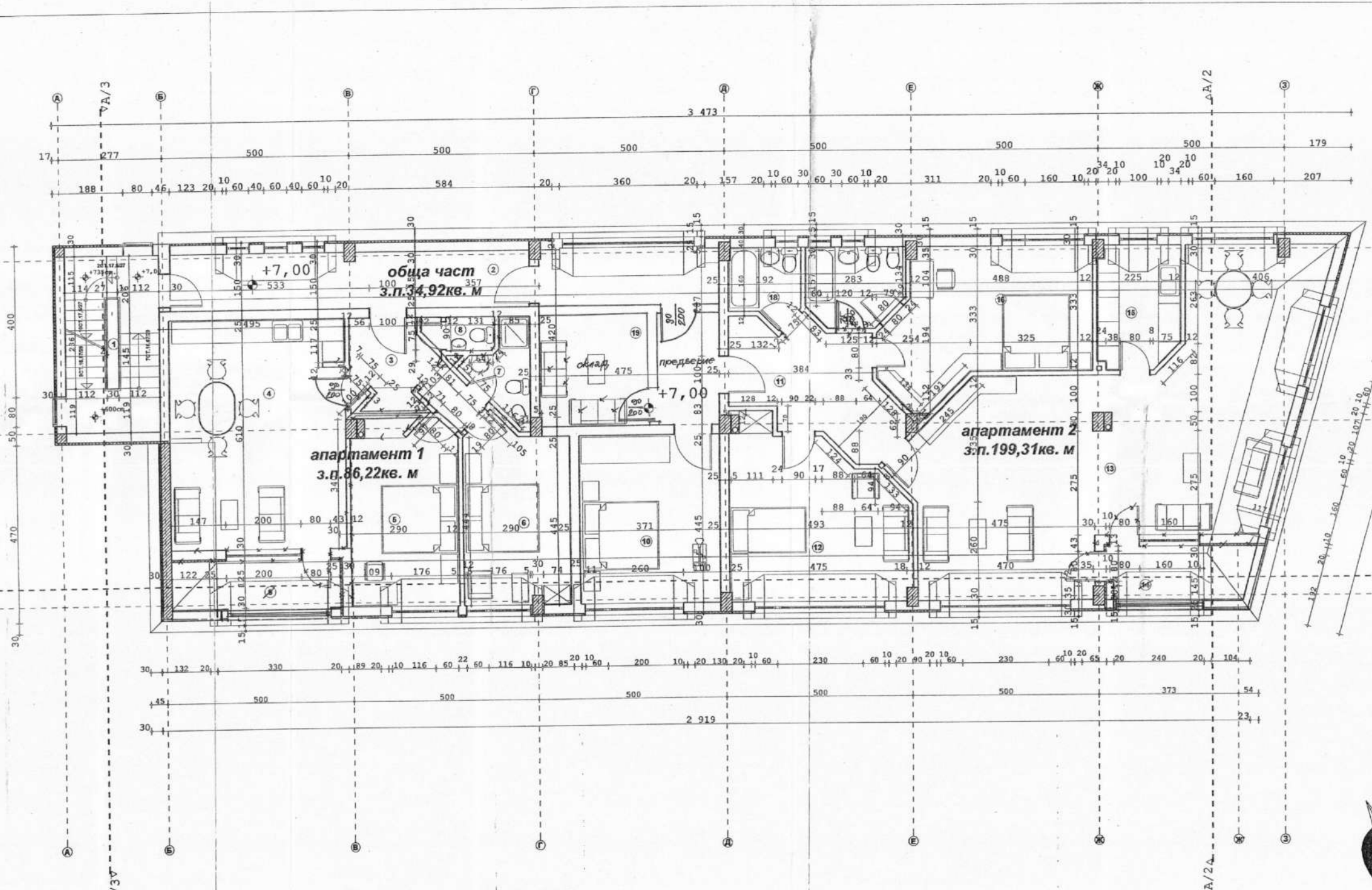
Разделение на кота +7.00 М 1:50
