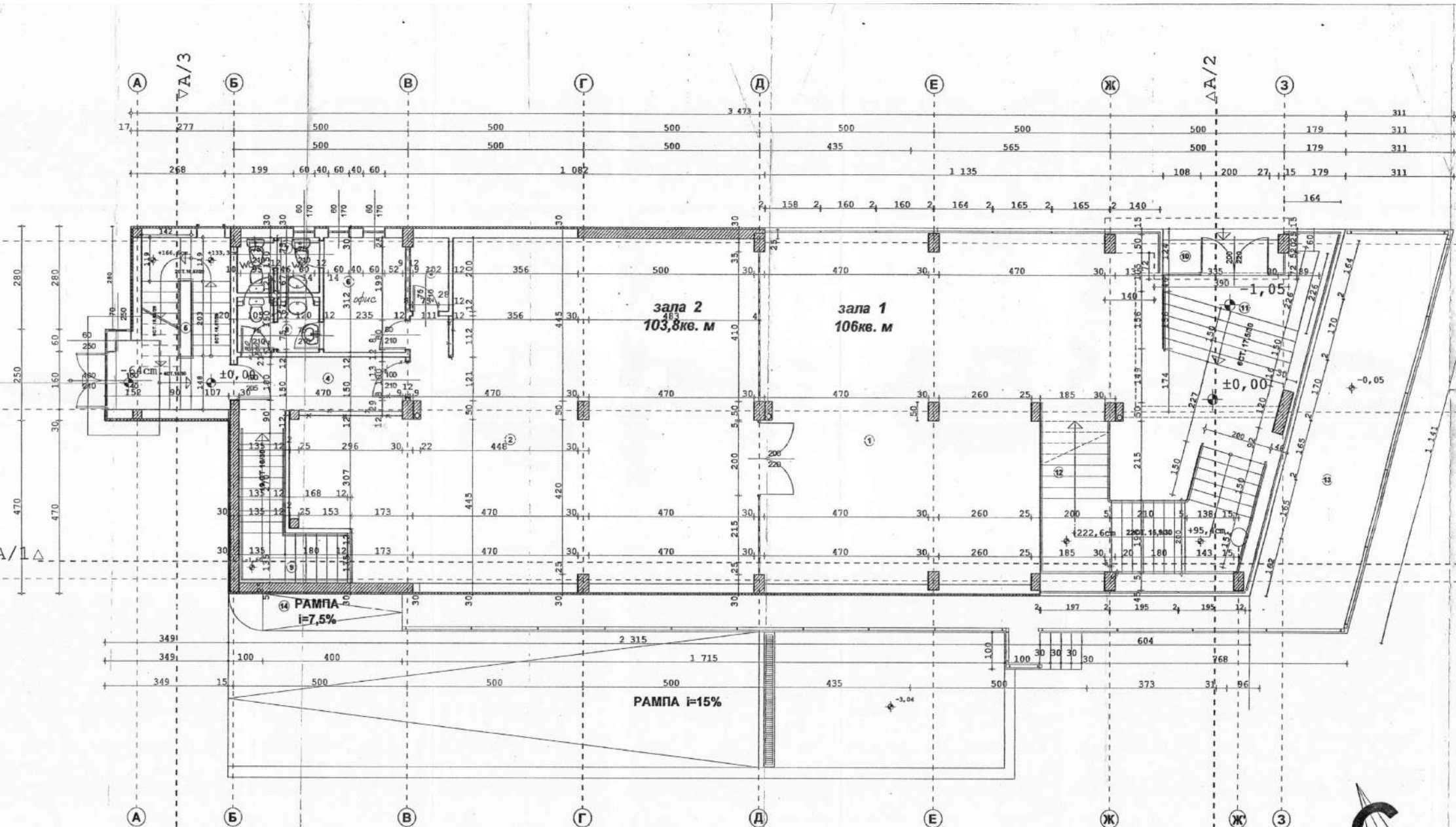
Разпределение на кота \pm 0.00 М 1:50
